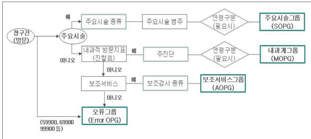
그림 1. KOPG 분류과정
