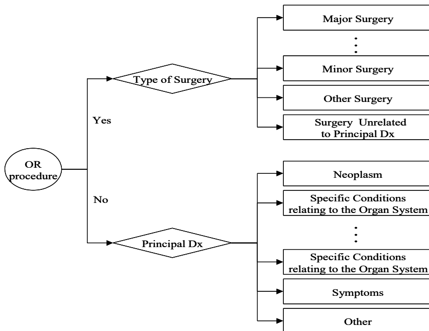
그림 2. ADRG 분류
