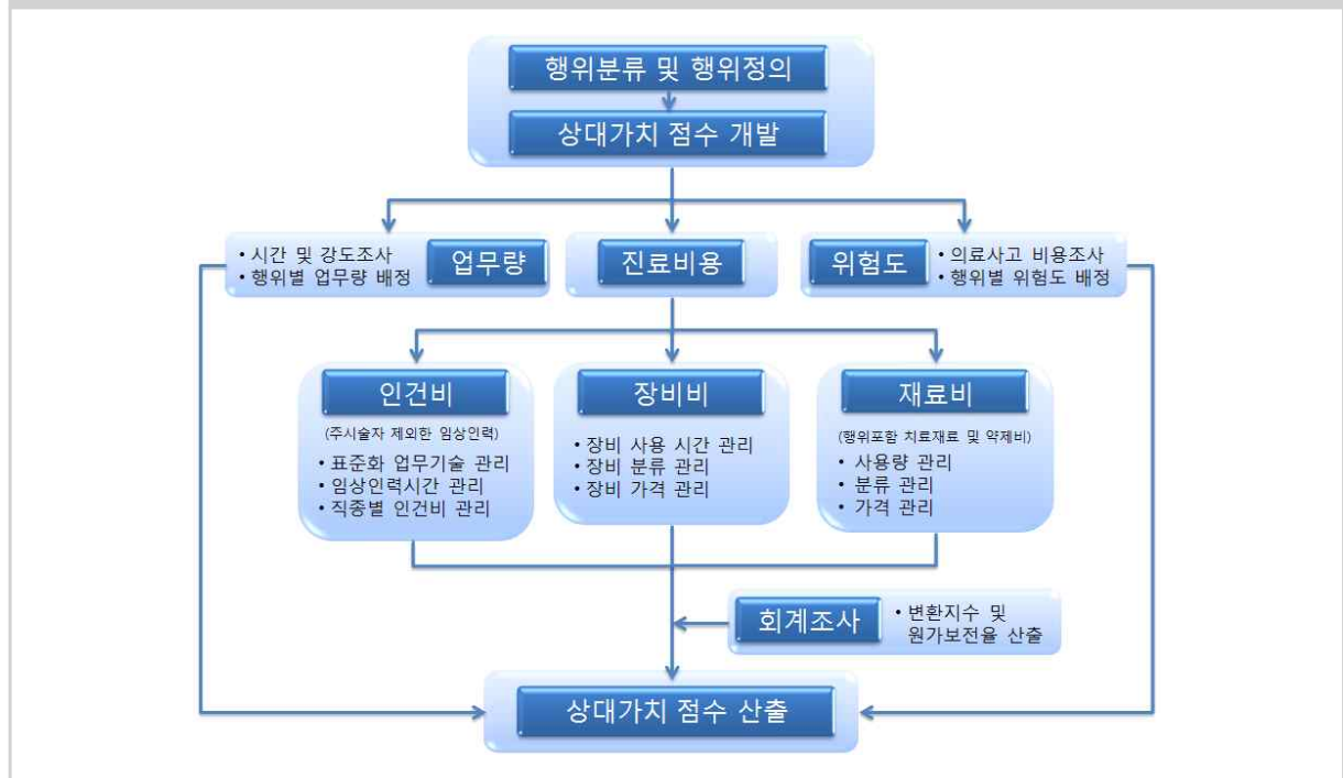
그림2.1-13 상대가치점수 개발 연구 산출 모형
